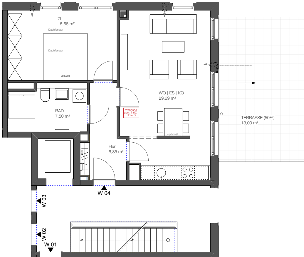
Erdgeschoss
